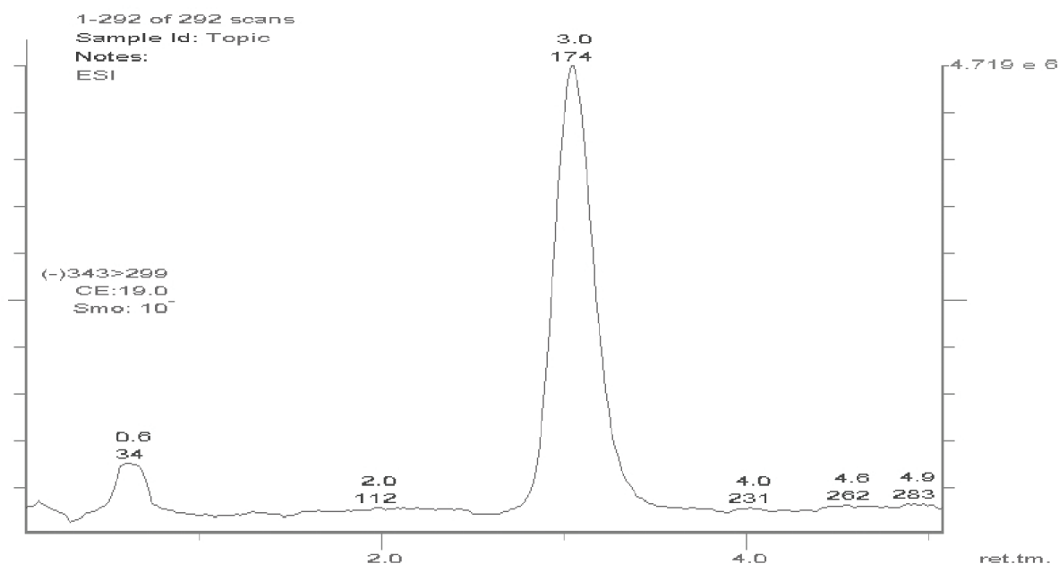
Obr. 3 LC-MS/MS spektrum získané nástřikem 15 \mu l vzorku moči pozitivní na přítomnost kanabinoidů, m/z 343 m/z 299.
