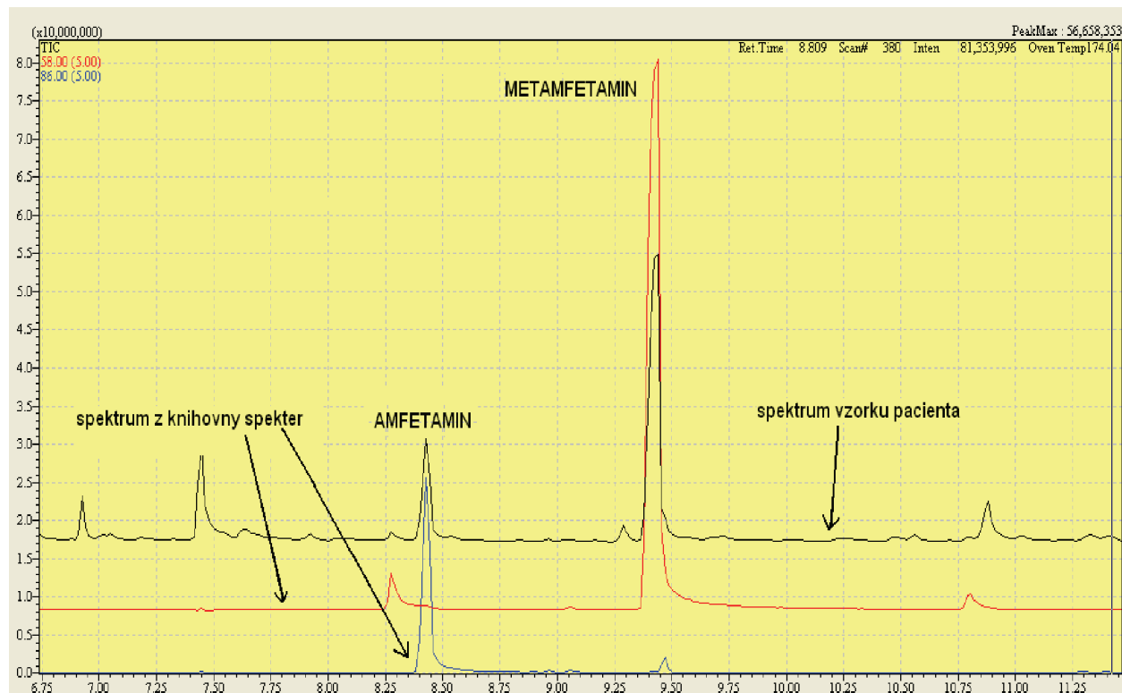
Obr. 2 Spektrum získané analýzou moče pozitivní na přítomnost amfetaminu a metamfetaminu metodou GC/MS. Spektrum získané analýzou moče pacienta je porovnáváno se spektry uloženými v knihovně spekter. Na obrázku je shoda píku amfetaminu a metamfetaminu ve spektech z knihovny spekter a ve spektru pacienta. Jedná se o vzorek, který byl nanesen na TestCard, viz obr. 1.
