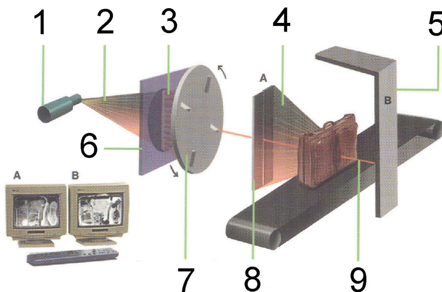
Popis obrázku č. 1 – Schéma rentgenového systému AS&E
